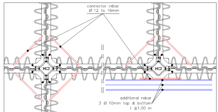
X ja T-liitososa, mustissa pisteissä asennushitsaus
